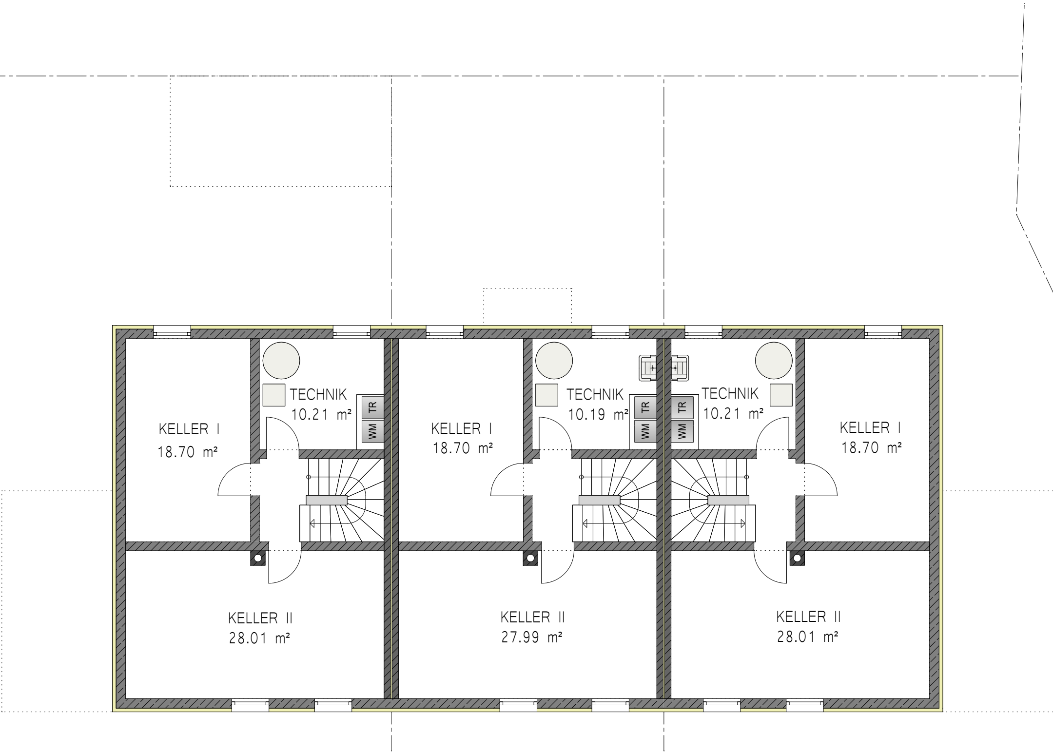
KELLERGESCHOSS
