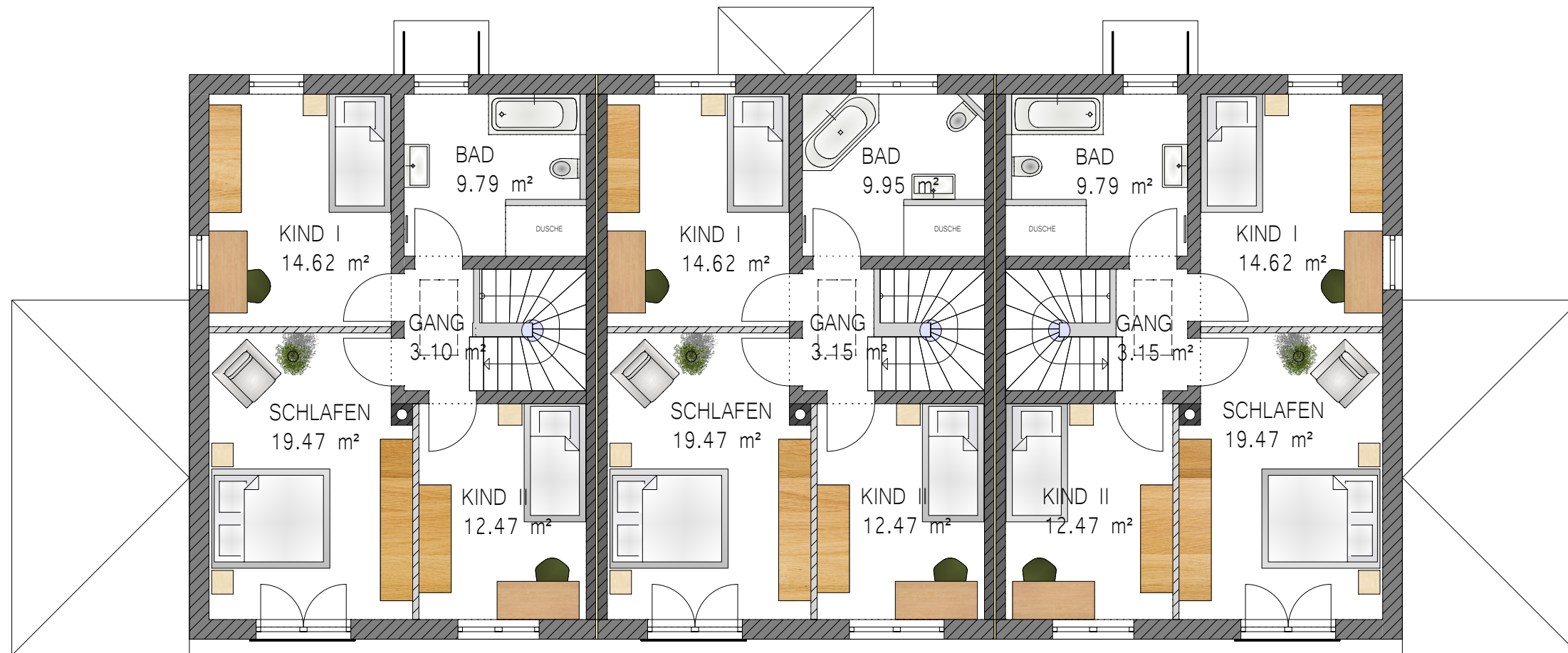
OBERGESCHOSS
